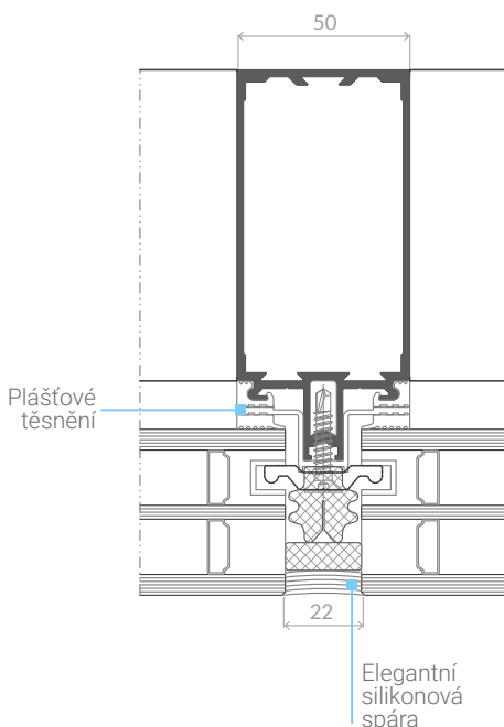
Řez sloupku
